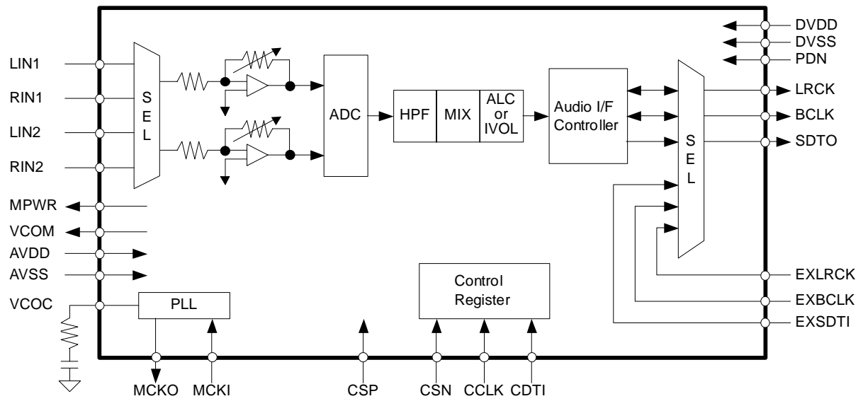
Figure 1. ブロック図
