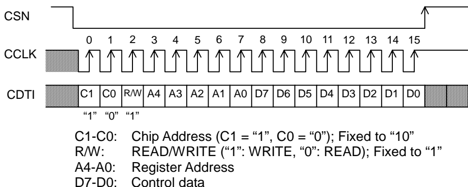
Figure 41. シリアルコントロールインタフェースタイミング(CSP pin = “L”)
