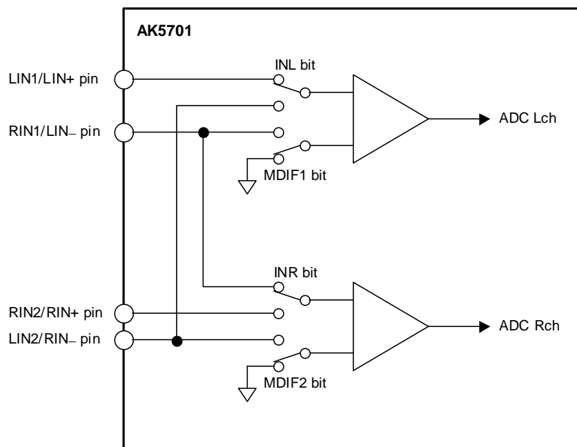
Figure 36. マイク / ライン入力セレクト
