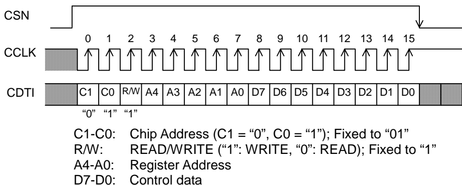
Figure 42. シリアルコントロールインタフェースタイミング(CSP pin = “H”)
