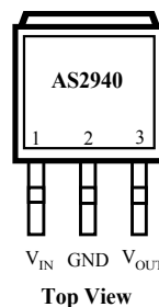
TO-263-3 (T)
