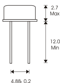
HC-49/SS
