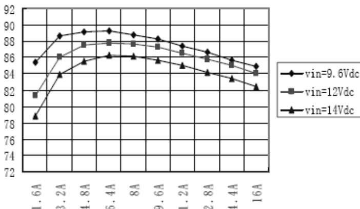
Vout 1.8V:
