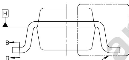
VIEW A-A
