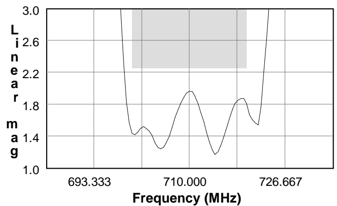
S11 VSWR
