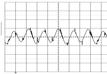
Trace: output voltage (20mV/div.). Time scale: (2 \mu s/div.).
