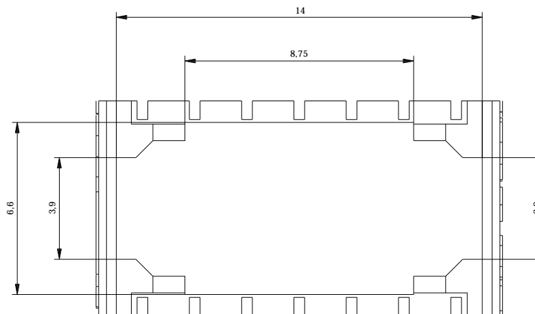
DETAIL X (10:1)
