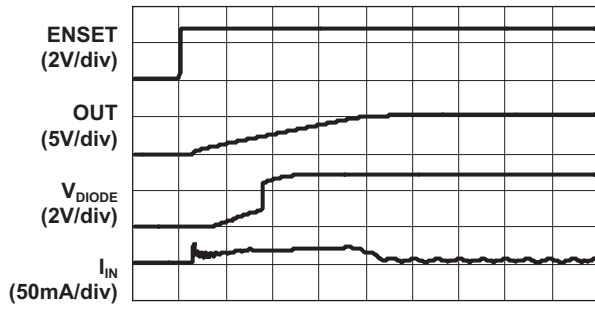
Turn-On
