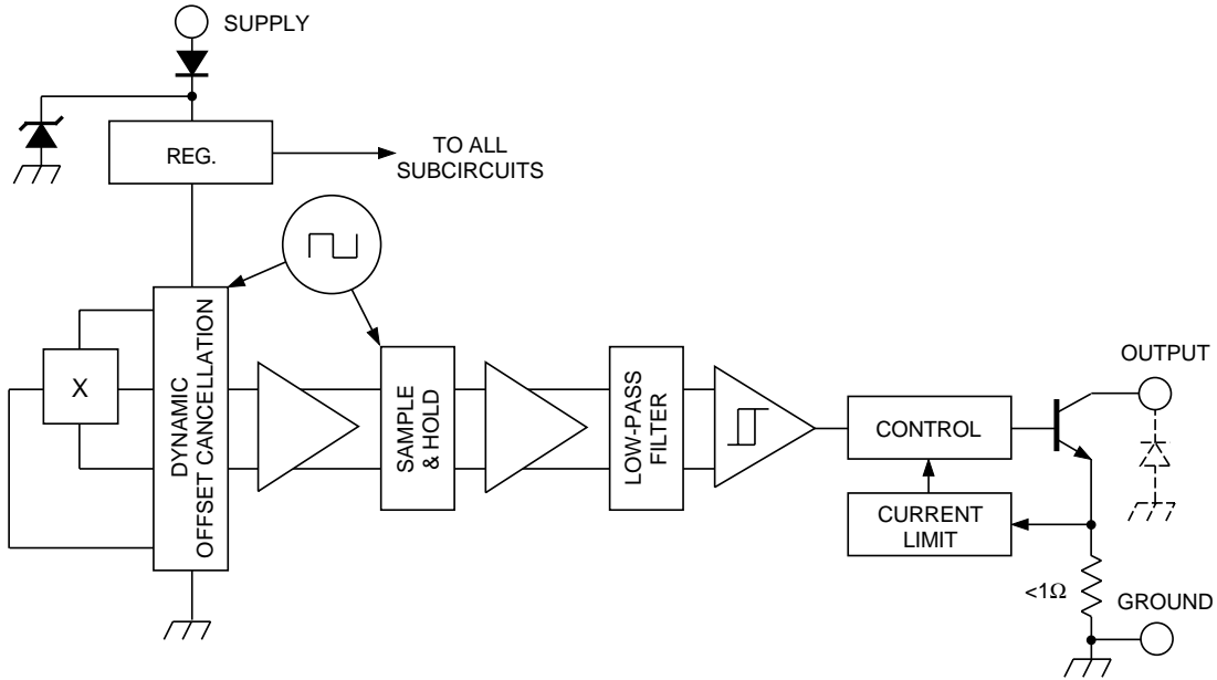
Dwg. FH-020-1
