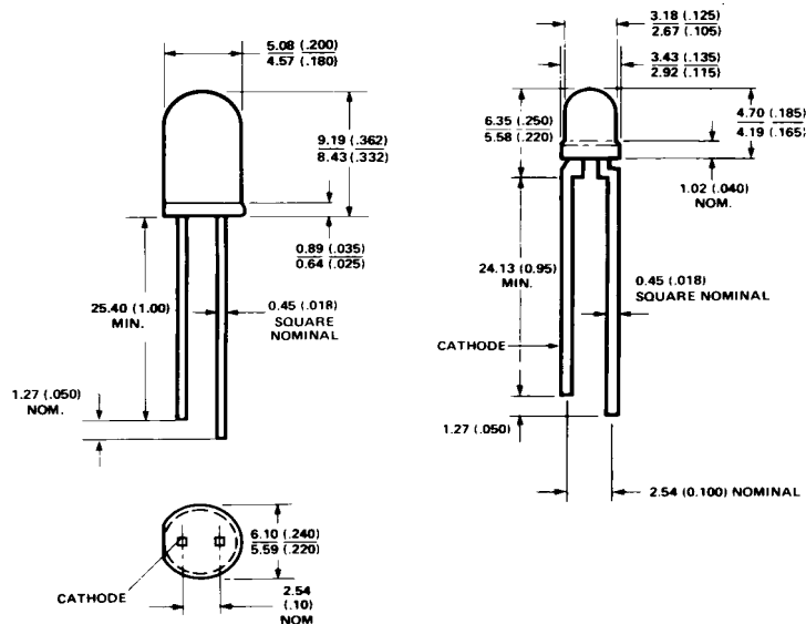
HLMP-4700, -4719, -4740
